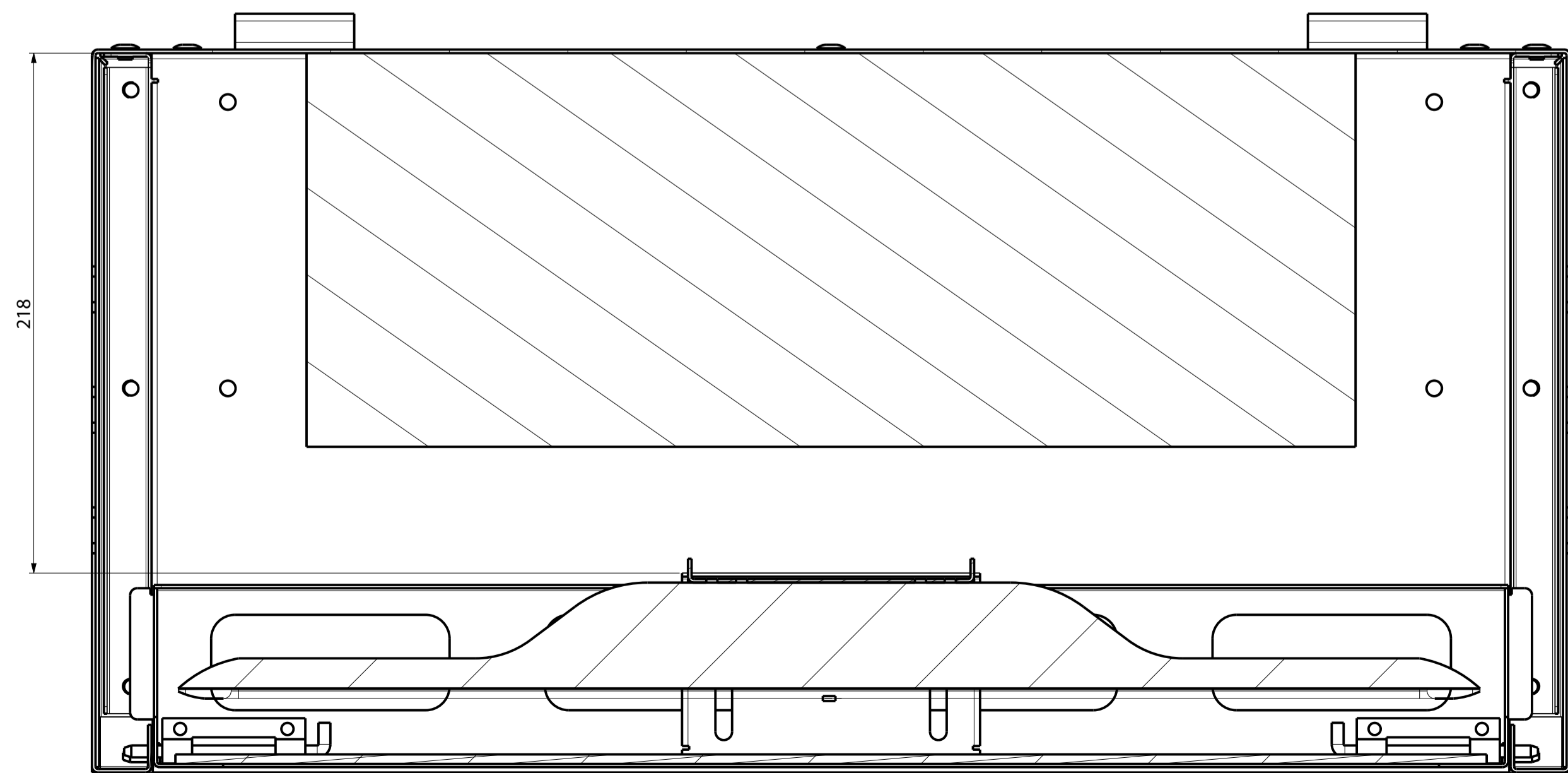
SEZIONE B-B
